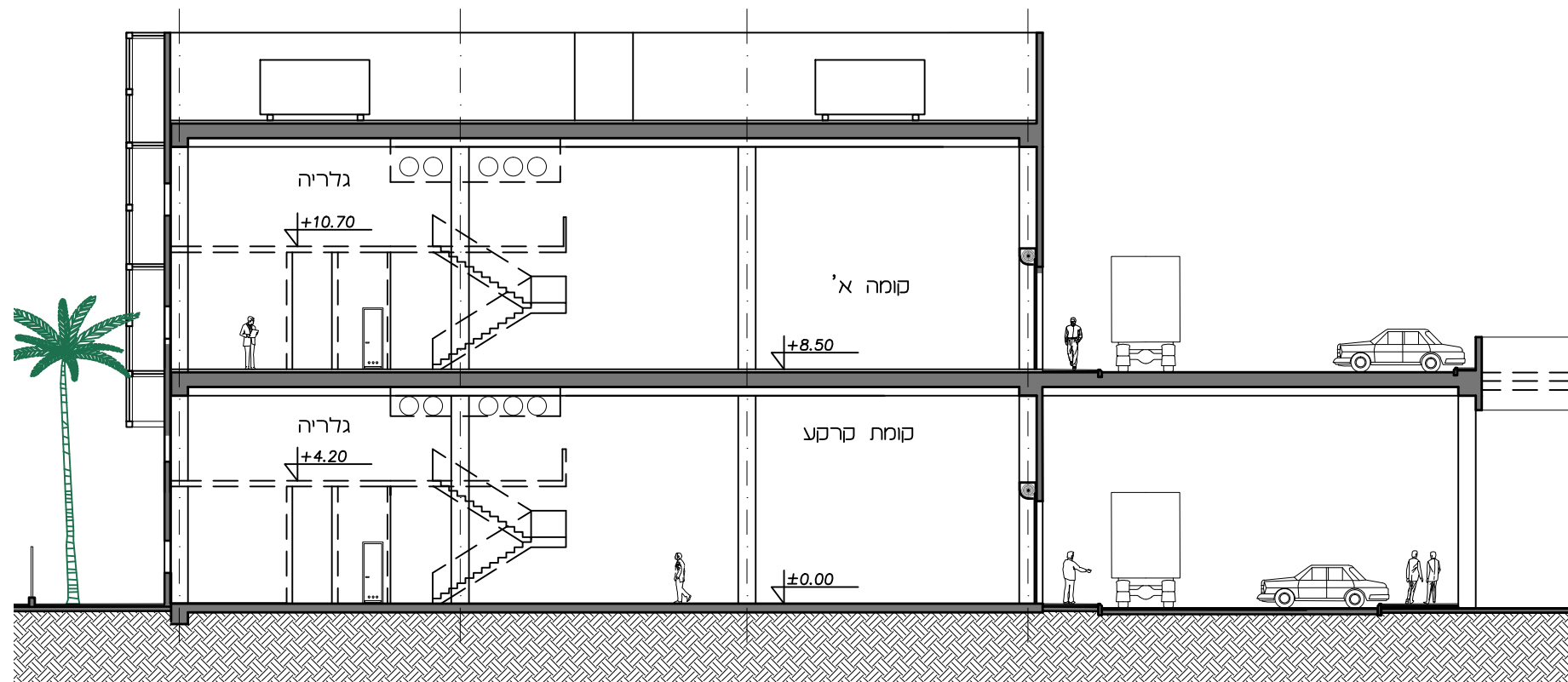
יחידה טיפוסית * חתך
